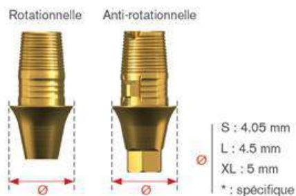
Figure 23- Représentation d'une Embase préfabriquée en titane. Document fourni par l'aimable contribution de Mr Cédric LANCIEUX, Directeur R&D et cad-cam de LYRA®
